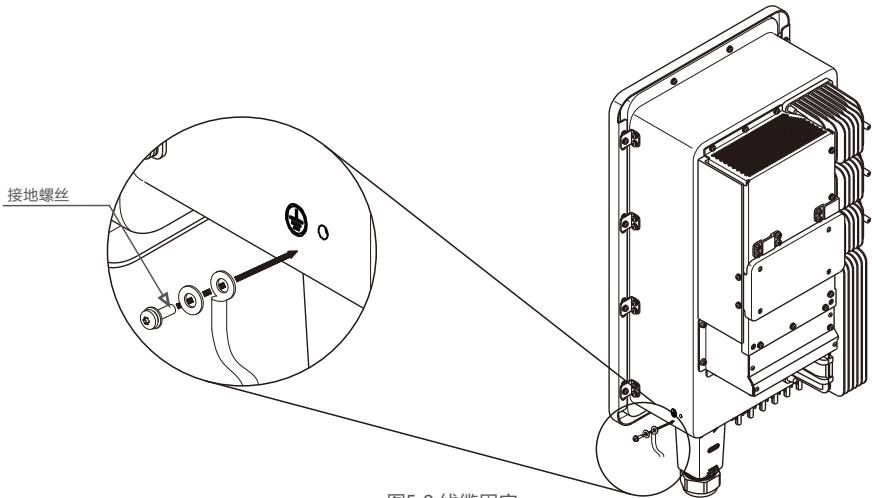
图5.9 线缆固定
