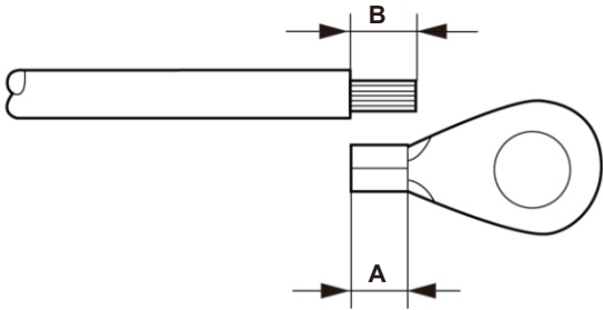
图5.7 剥线长度
