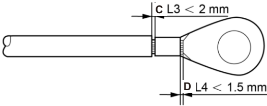
图5.8 线缆压接
